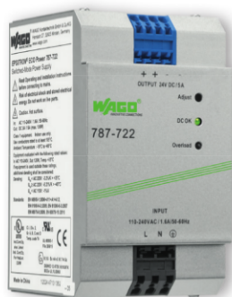
787-722 ECO Tápegység, 1-fázisú 24 VDC / 5 A
